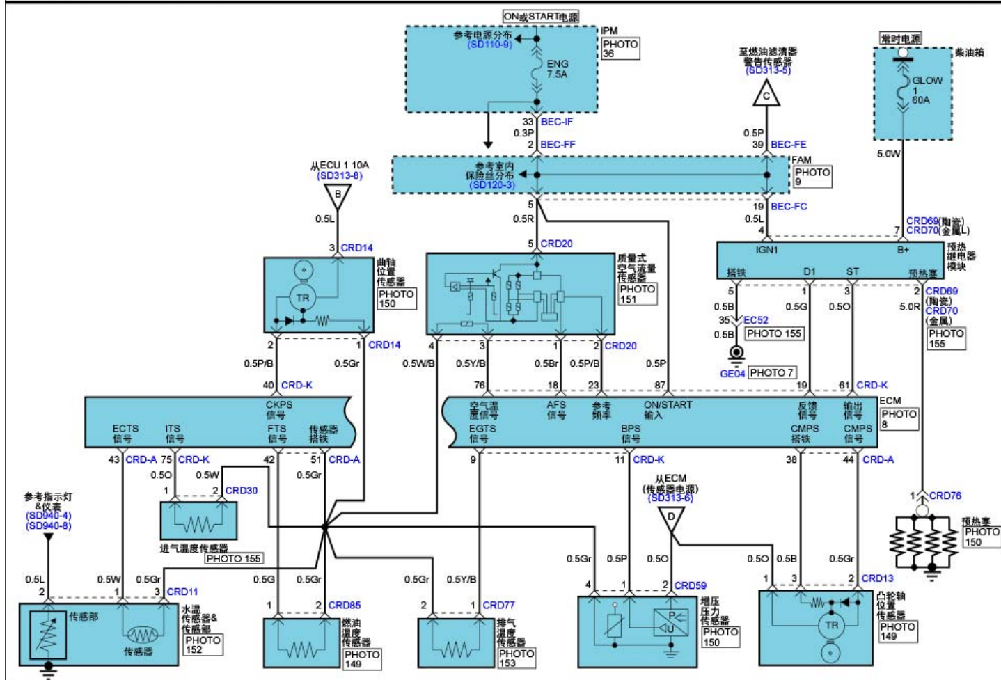
发动机控制系统(D4HB : R 2.2L)(4)
